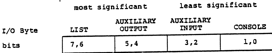
Figure 4-3. I/O Byte
